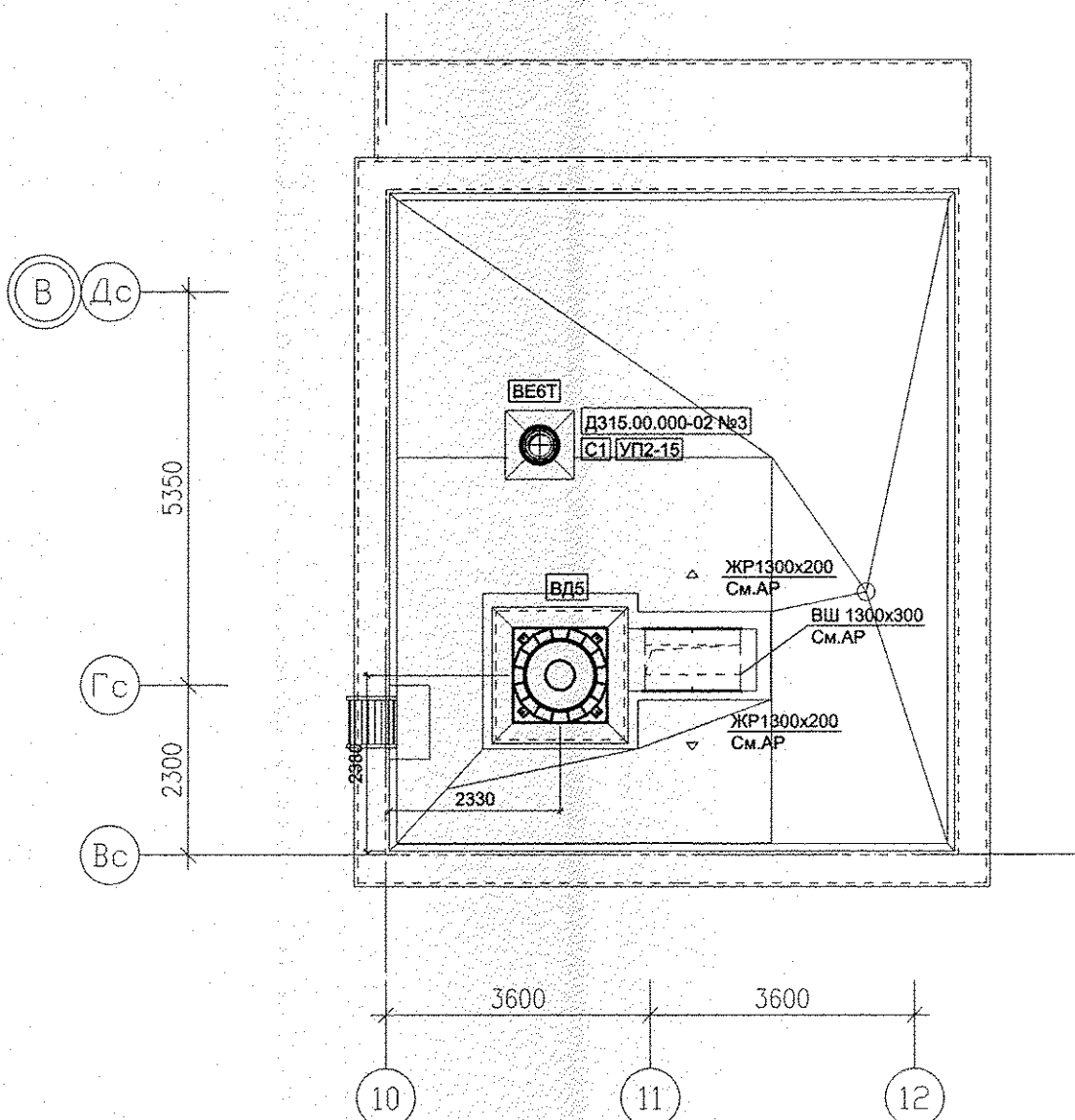
План кровли над машинным помещением
