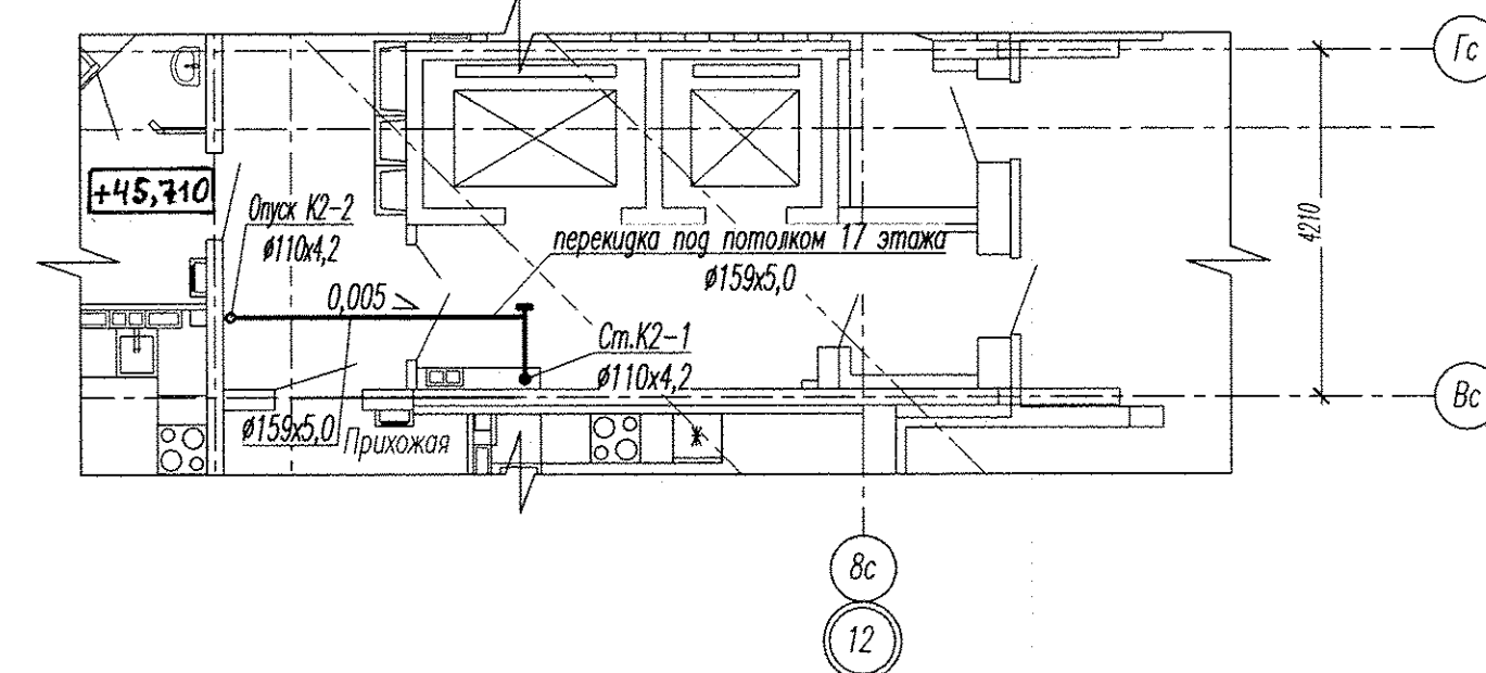
Фрагмент 2 плана 17 этажа в осях Гс-Вс.
