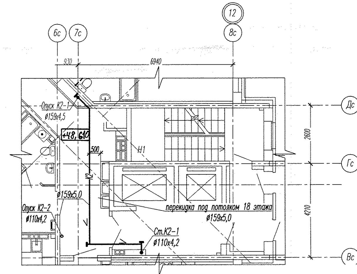
Фрагмент 1 плана 18 этажа в осях 6с-8с.
