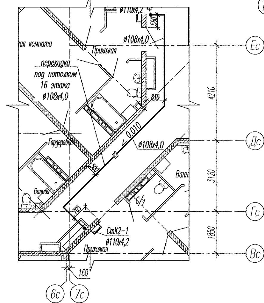
Фрагмент 1 плана 16 этажа в осях Ес-Вс.
