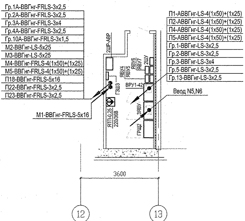
План расположения оборудования и питающих сетей в электрощитовой
