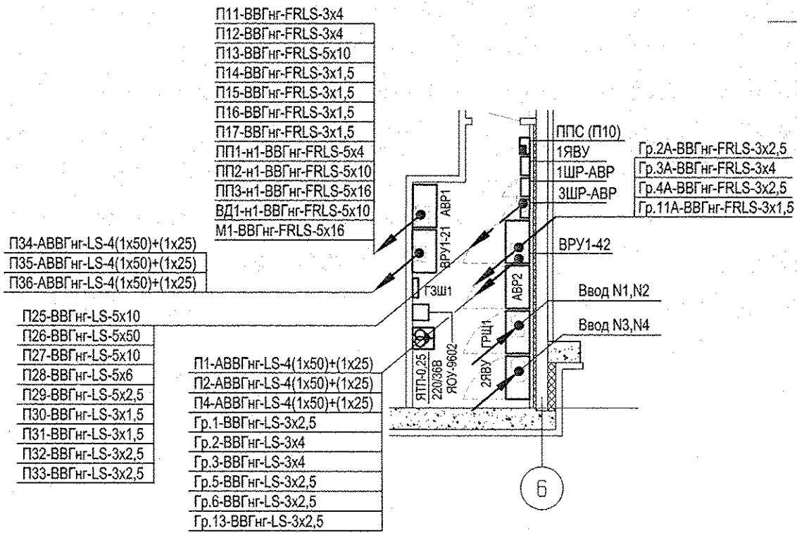
План расположения оборудования и питающих сетей в электрощитовой
