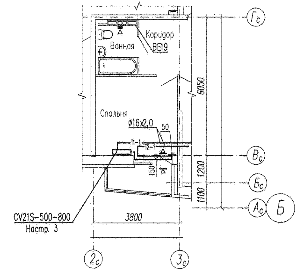
Фрагмент 2 План 16 этажа в осях 3-4 (2с-3с, Ас-Гс)
