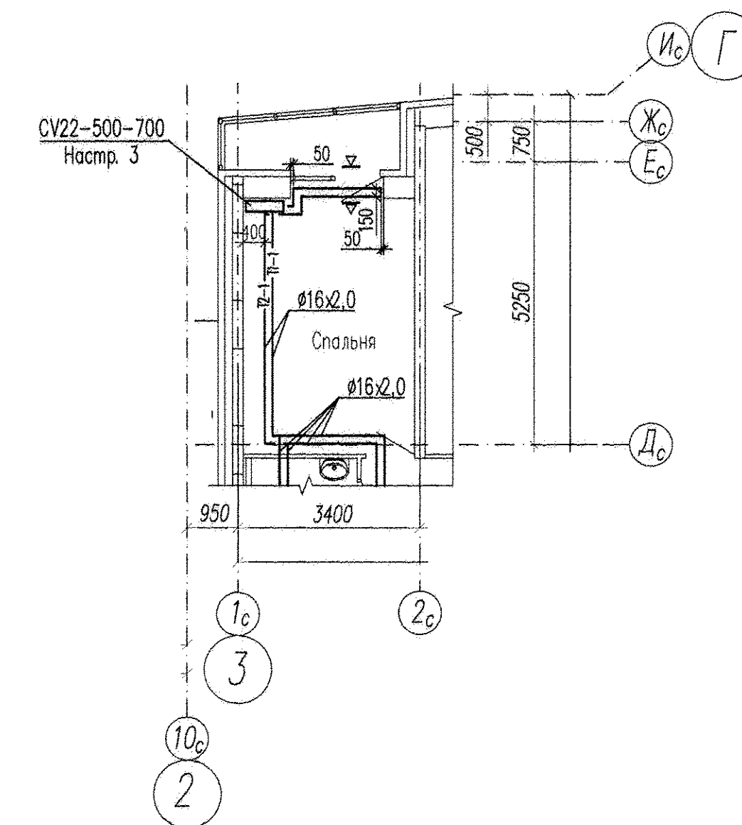
Фрагмент 1 План 16 этажа в осях 3-4 (1с-2с, Дс-Ис)
