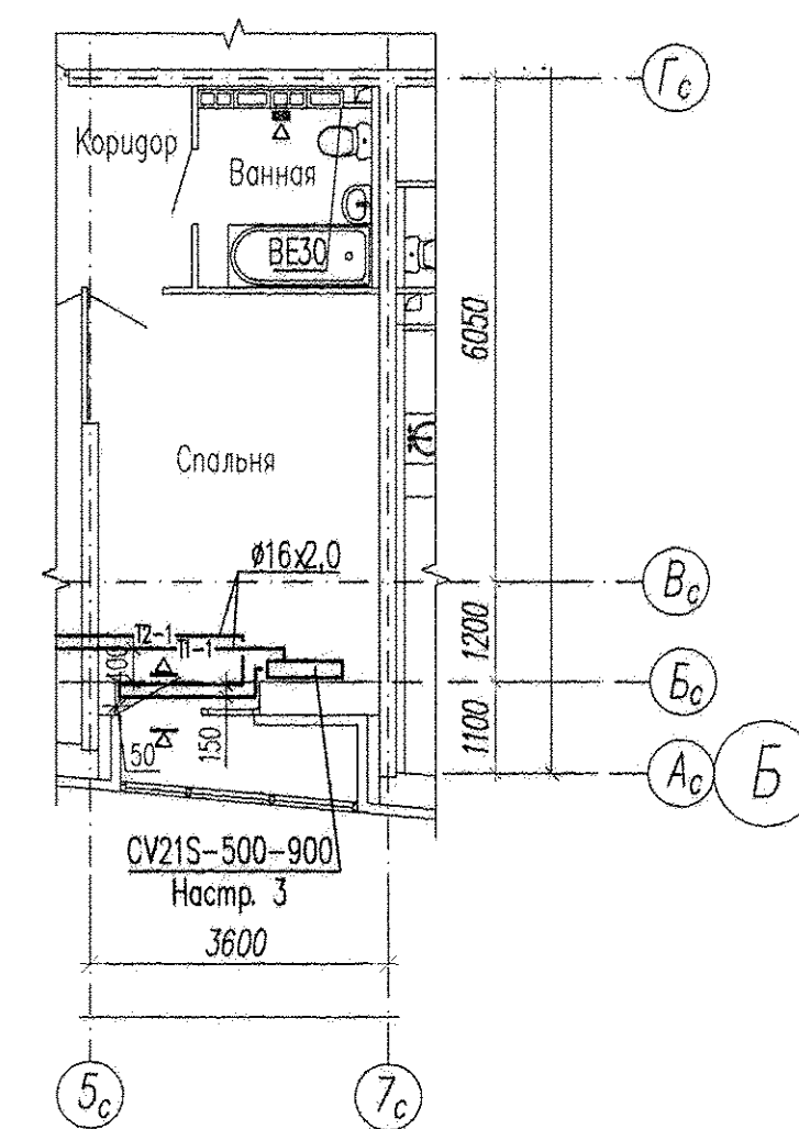
Фрагмент 3 План 16 этажа в осях 3-4 (5с-7с, Ас-Гс)
