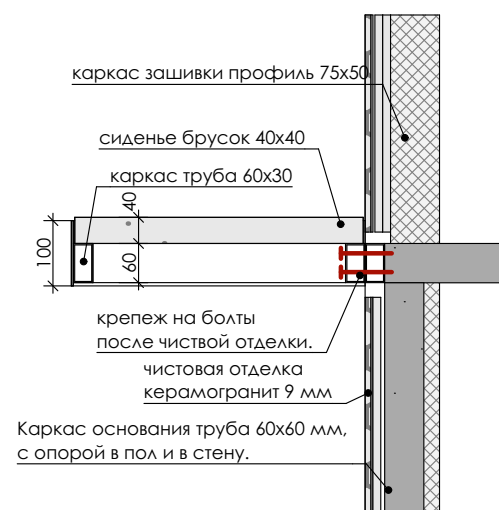
Узел монтажа скамейки
