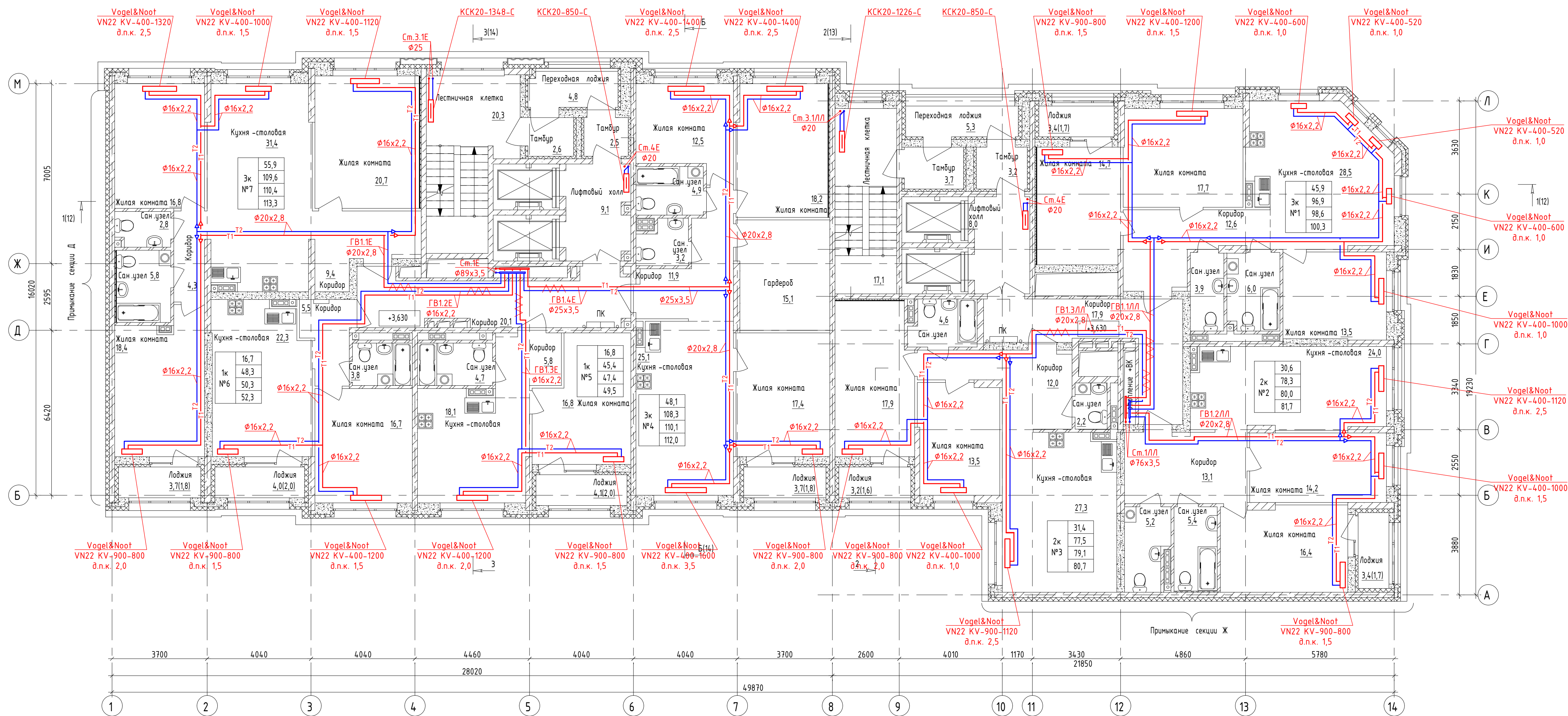
План на отм. +3.630 (2 этаж)
