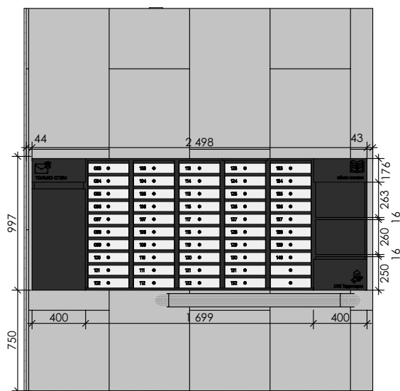
Вид М01 (вид спереди)
