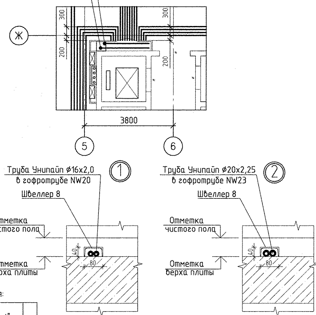
Фрагмент плана 17-го...20-го этажей
