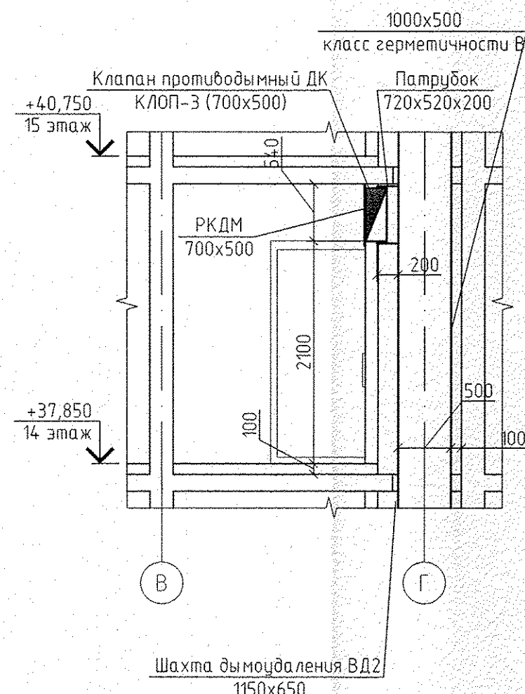
3-3 (М 1:50)
