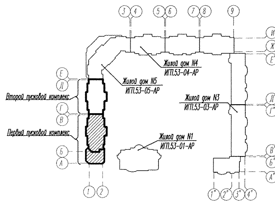
Компоновочная схема
