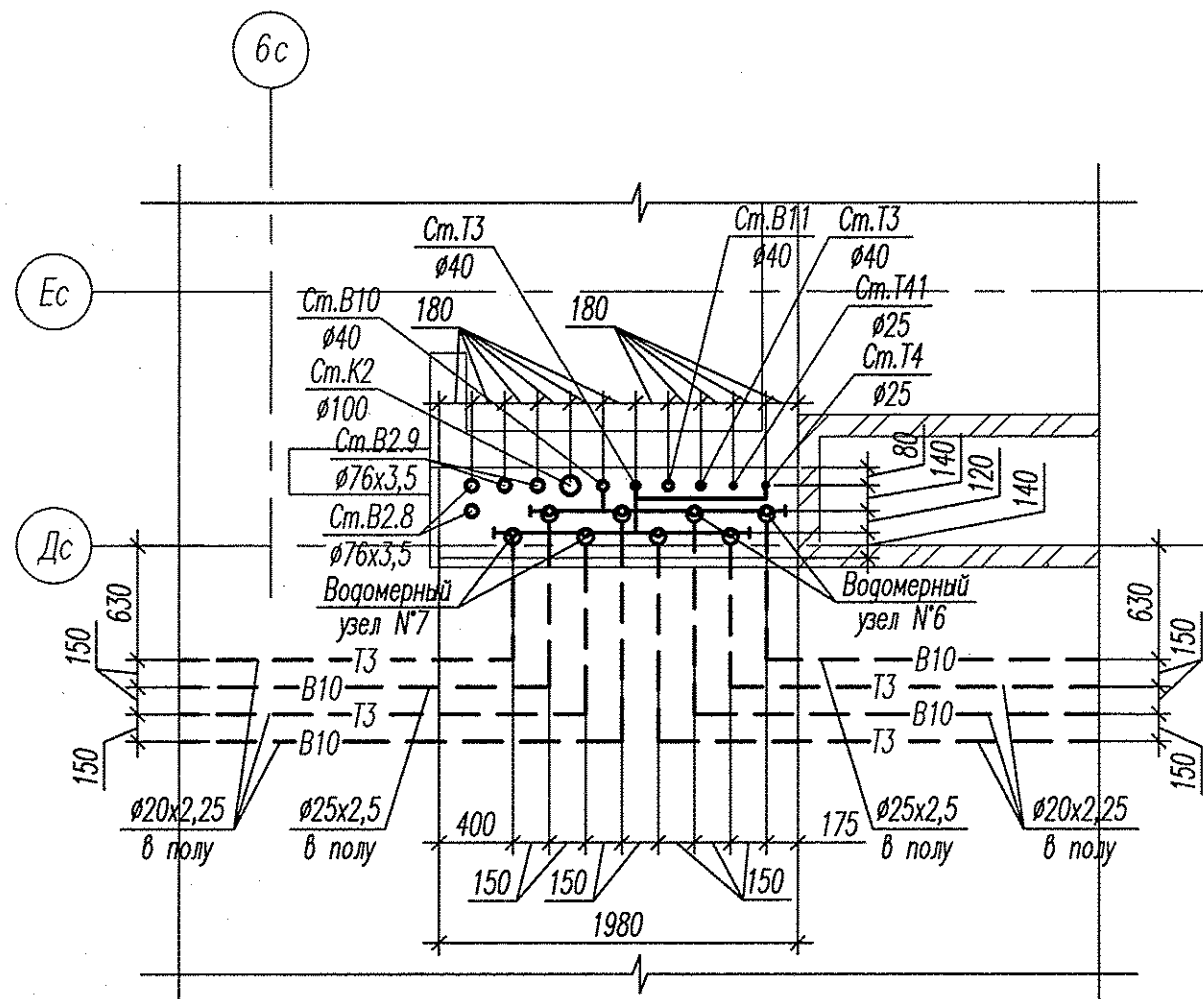
План размещения квартирных водомерных узлов в общей нише
