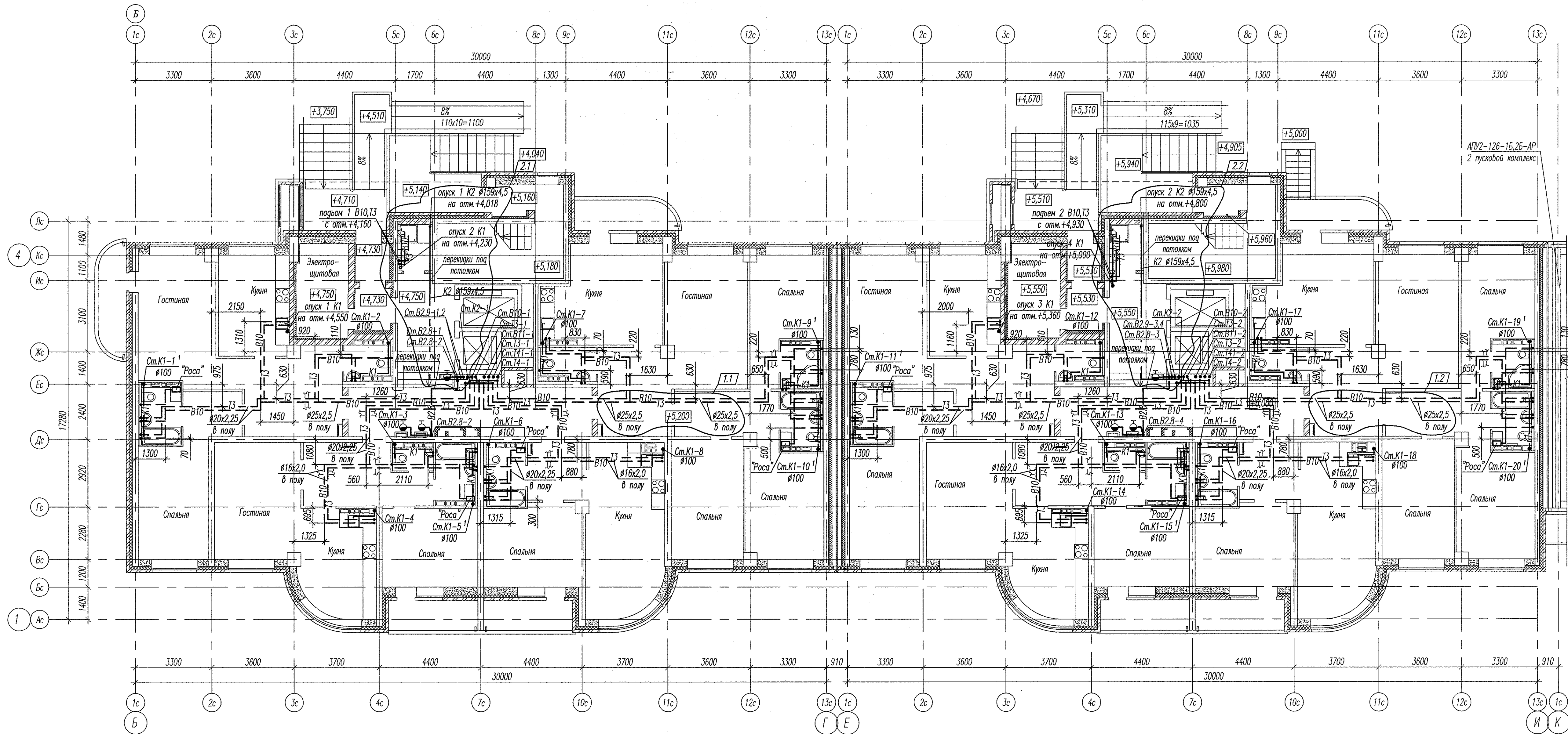
План 1 этажа
