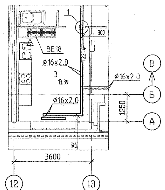
Фрагмент плана 12 этажа в осях 12-13/Б-В (1:100)
