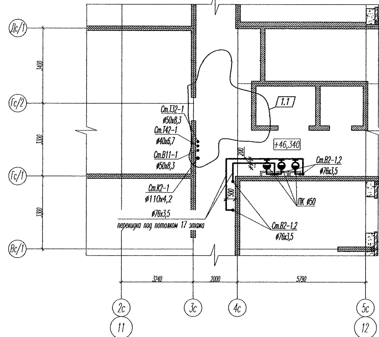
Фрагмент 1 плана 17 этажа в осях Дс/1-Вс/1.
