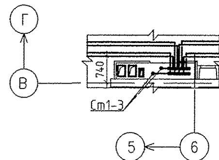
Фрагмент плана 8 этажа
