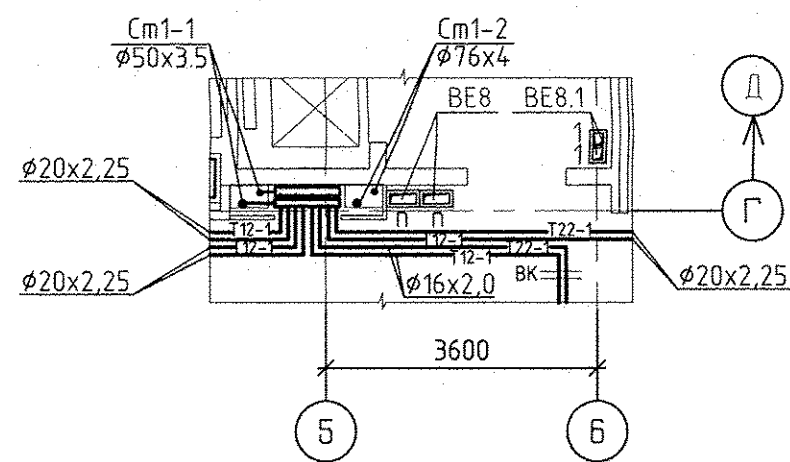
Фрагмент плана 6 этажа в осях 5-6/Г (1:100)
