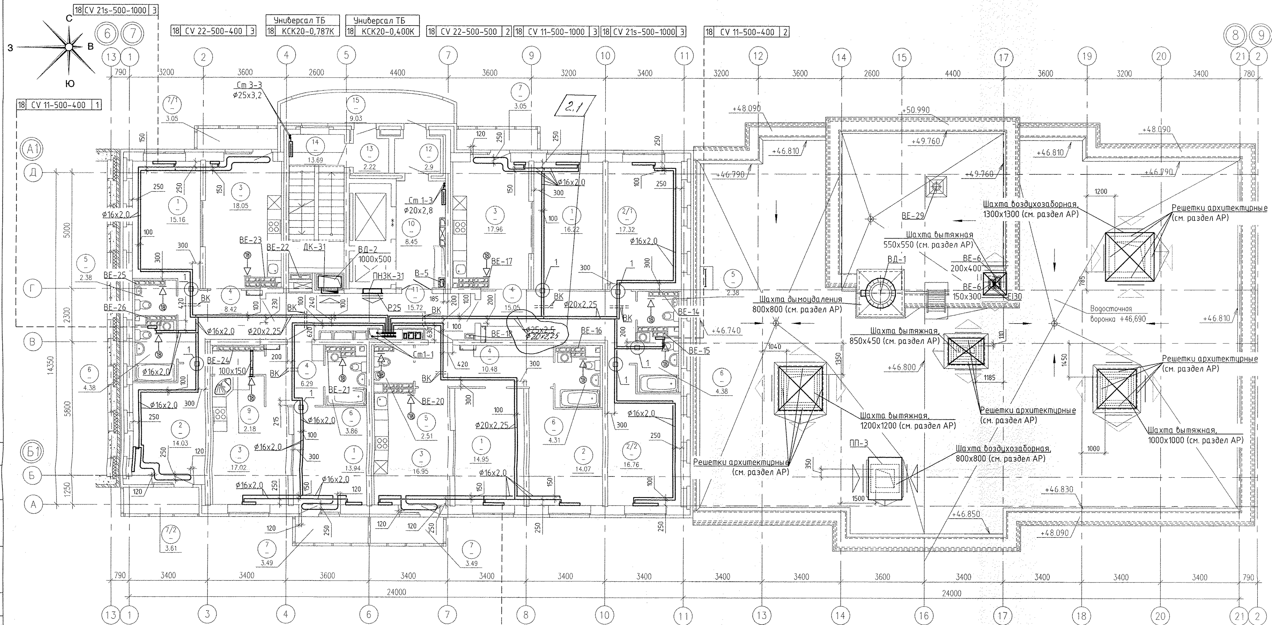
Экспликация помещений
